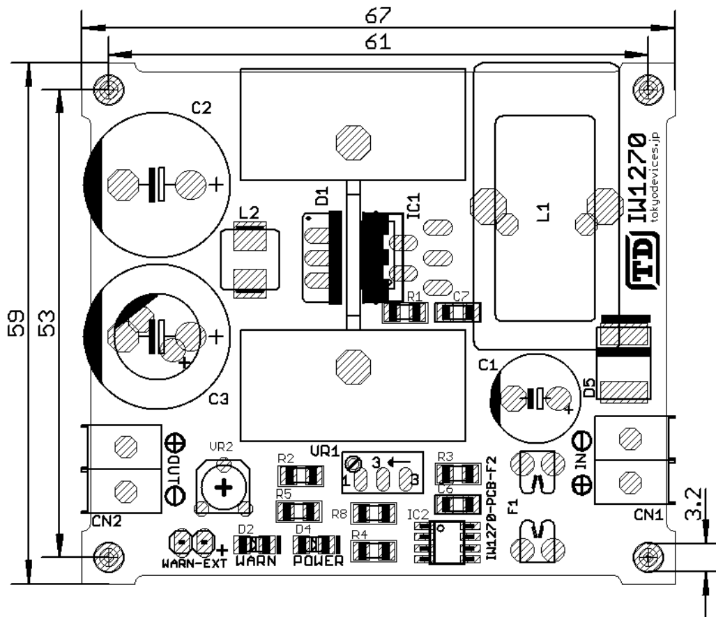
図 1 IW1270-X5 基板構成図
